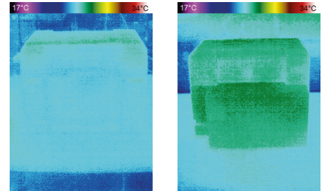
Vorder- und Rückseite des Epson SL-D800
