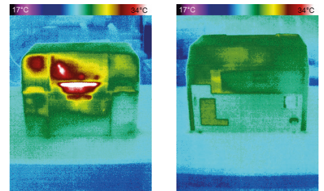
Vorder- und Rückseite eines Vierfarb-Tintenstrahldruckers der Konkurrenz
